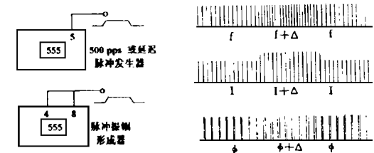
(b)实现调频、调相及 (c)电信号时域波形示意图 调幅的集成电路接法
